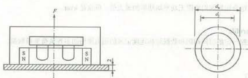
a) 吸力, 磁力线方向: N 极轴线指向多功能电能表 b) 尺寸: 内径 d_1=13\text{mm}\pm 1\text{mm} , 外径 d_2=28\text{mm} (最小值)
