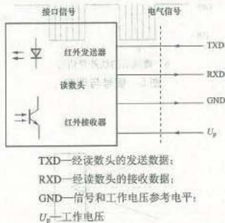
图 4 读数头的电气特性
