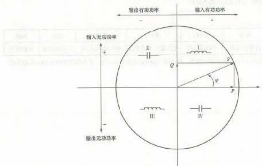
图 D.1 有功和无功功率的几何示意图
