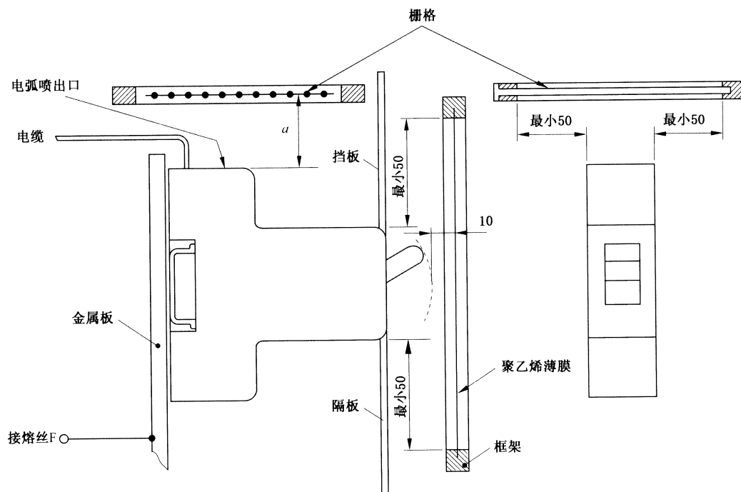
图 C.1 试验装置
